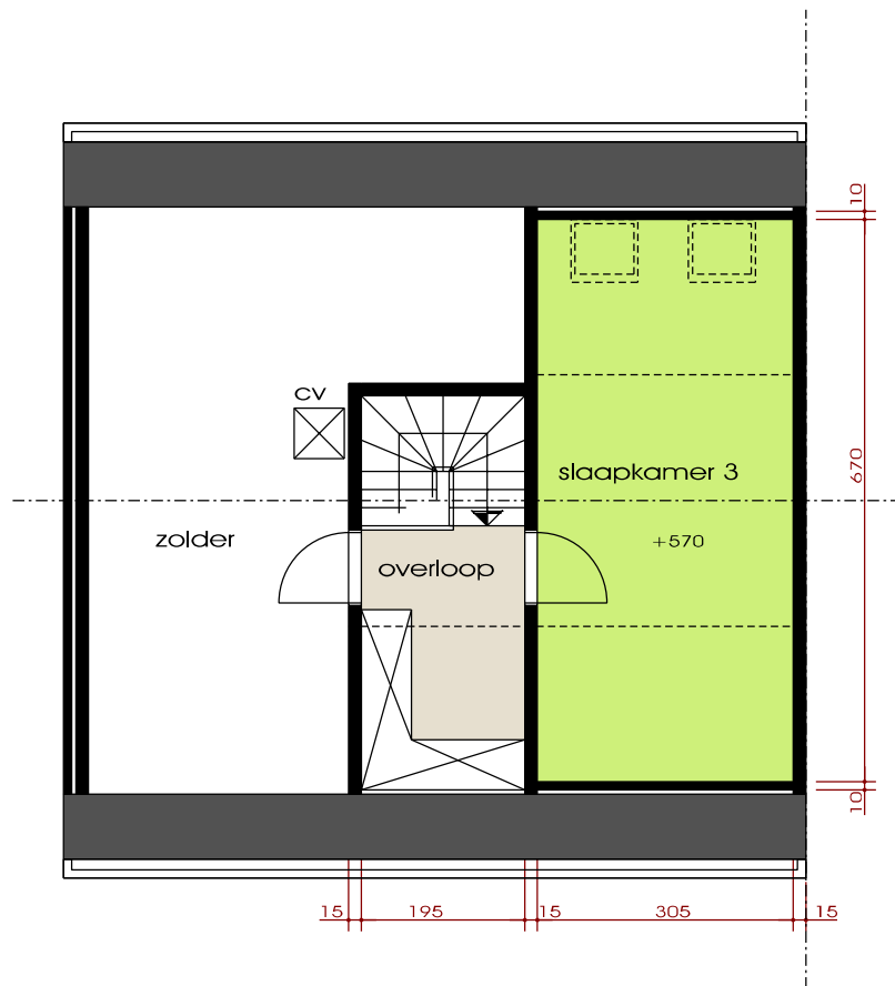
Dakverdieping
