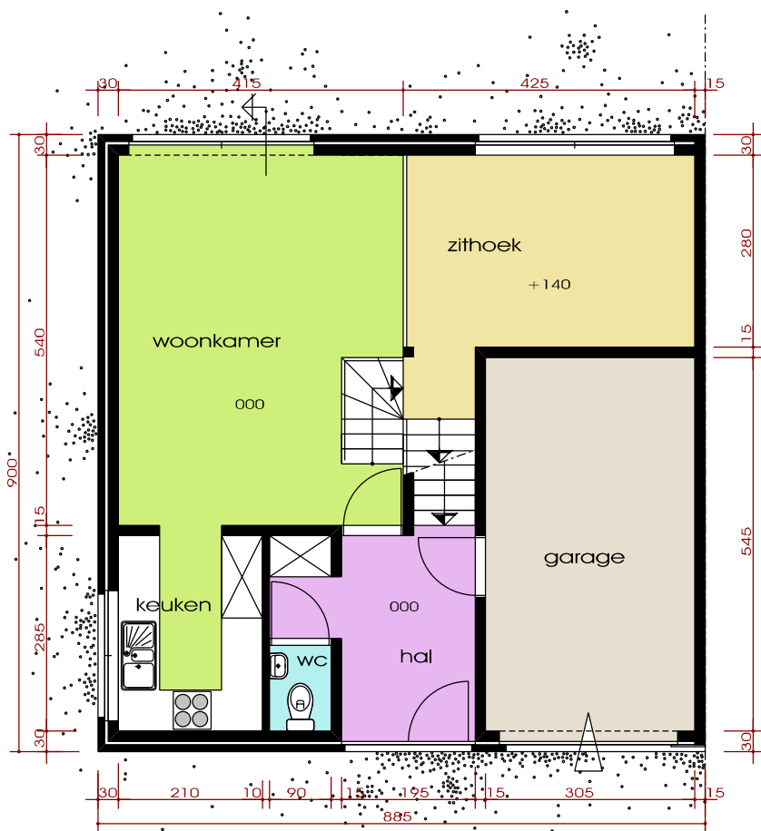
Gelijkvloers
