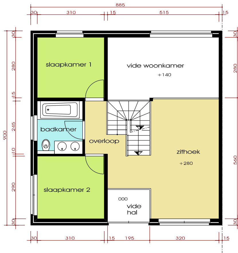
Verdieping
