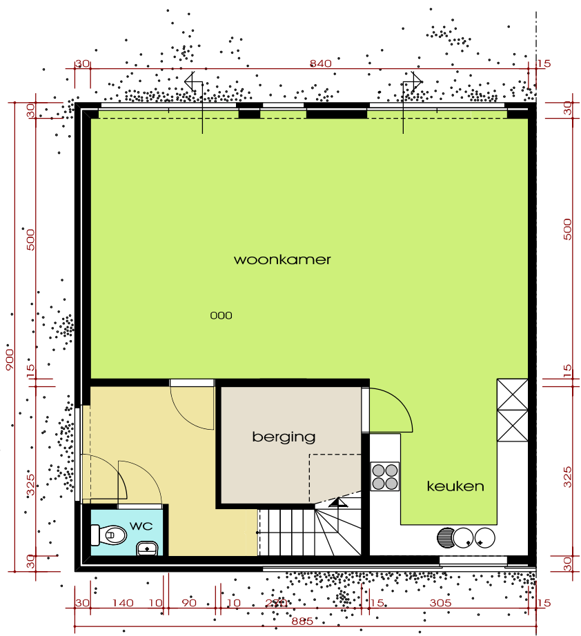
Gelijkvloers
