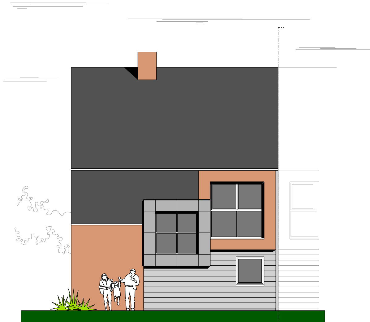
Voorgevel
